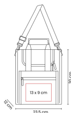
Área de impresión / Trazo técnico
